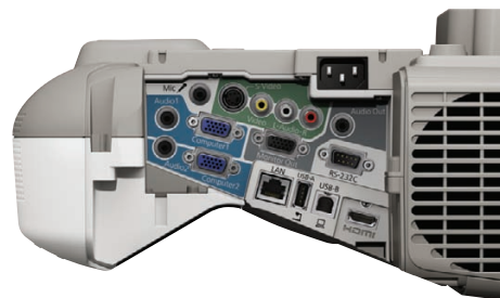
Rozhraní projektoru EB-485Wi
